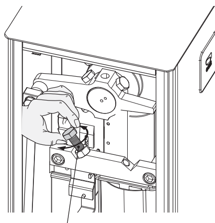
Fermo meccanico
