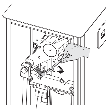
Controdado
