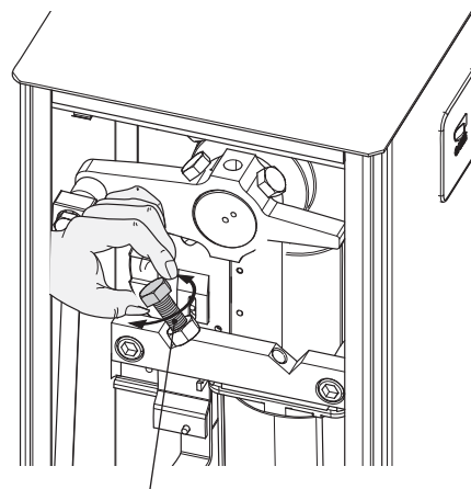
Механический упор
