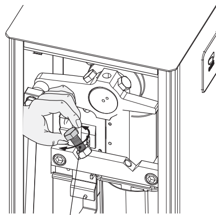
Butée mécanique
